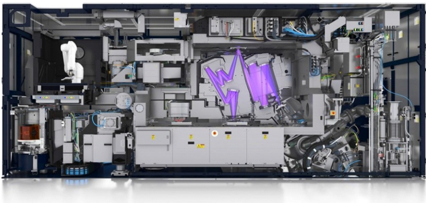
图1 EUV光刻内部结构图
