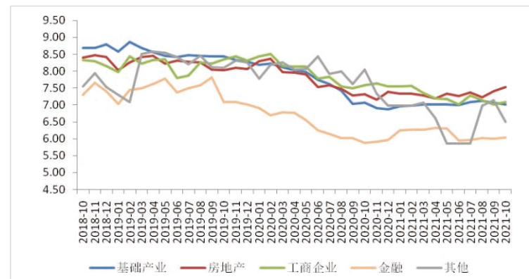
图4 2018年10月-2021年10月信托产品投向成立收益率 (%)
