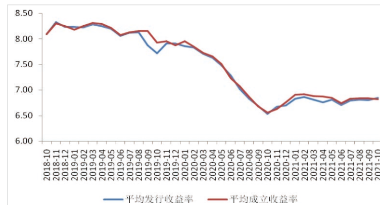
图4 2018年10月-2021年10月信托产品投向成立收益率 (%)
