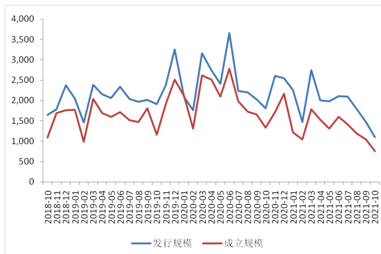
图1 2018年10月—2021年10月信托产品发行规模与成立规模（亿元）
